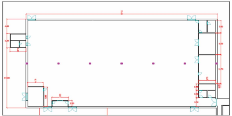
a főépület alaprajza
