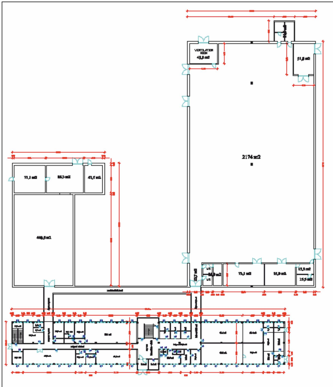
az építmény részletes alaprajza
